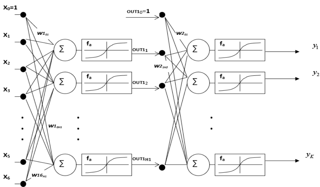
Рис. 2. Структура персептрона с одним скрытым слоем
